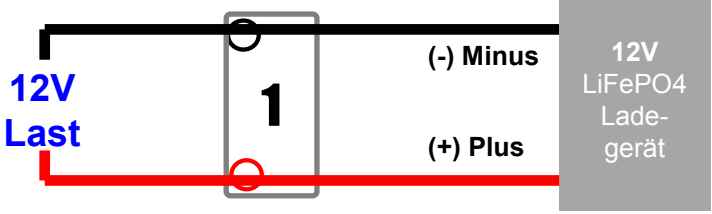
12V Anschluss / Single Batterie
